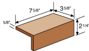
EDGE CAP
